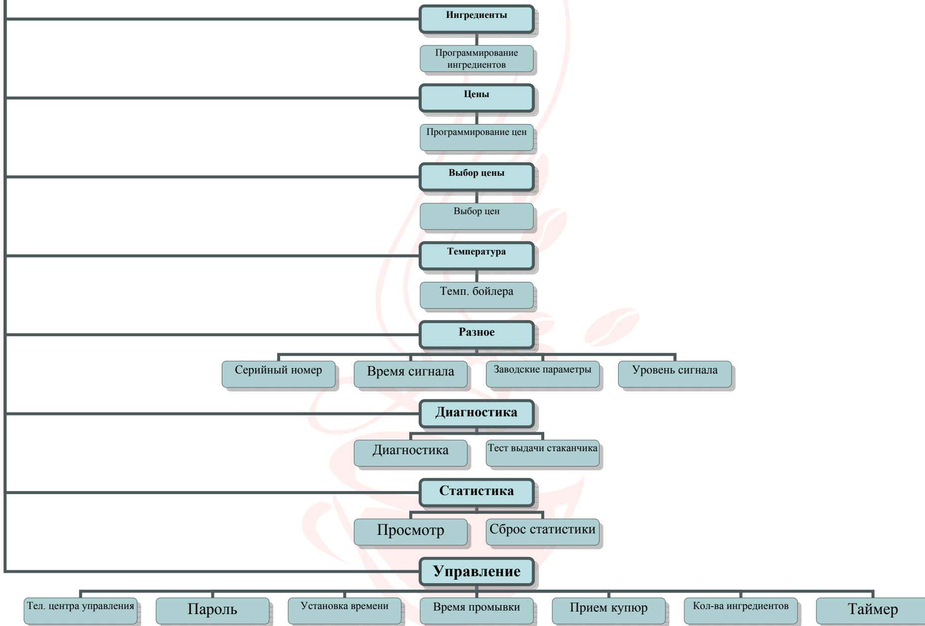
Рис. 10 Структура меню в режиме «Программирование»
