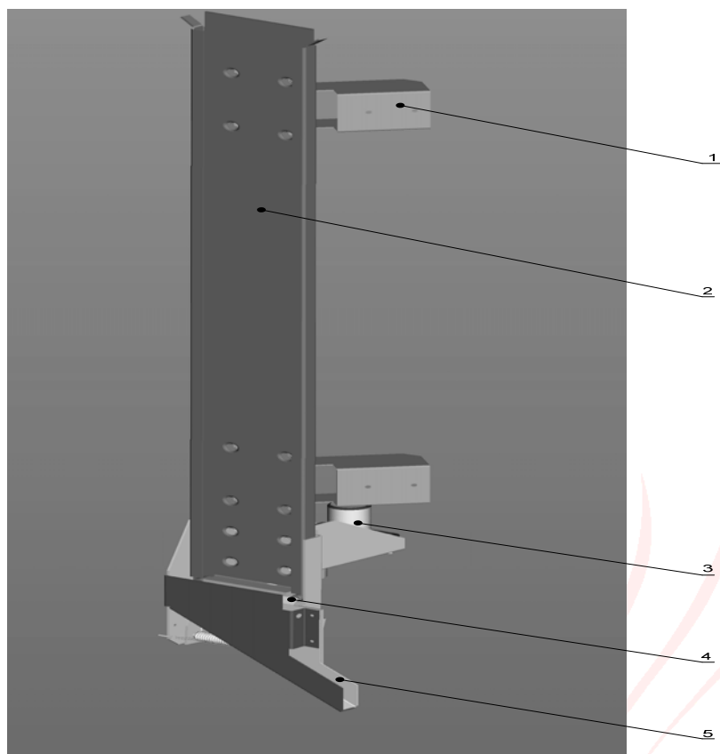
Рис.6. Блок выдачи палочек.
