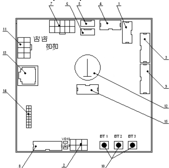
Рис. 8. Процессорная плата
