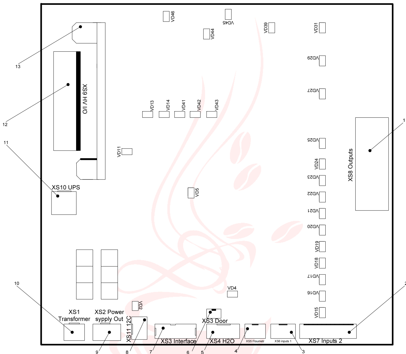
Рис. 7. Плата автоматки
