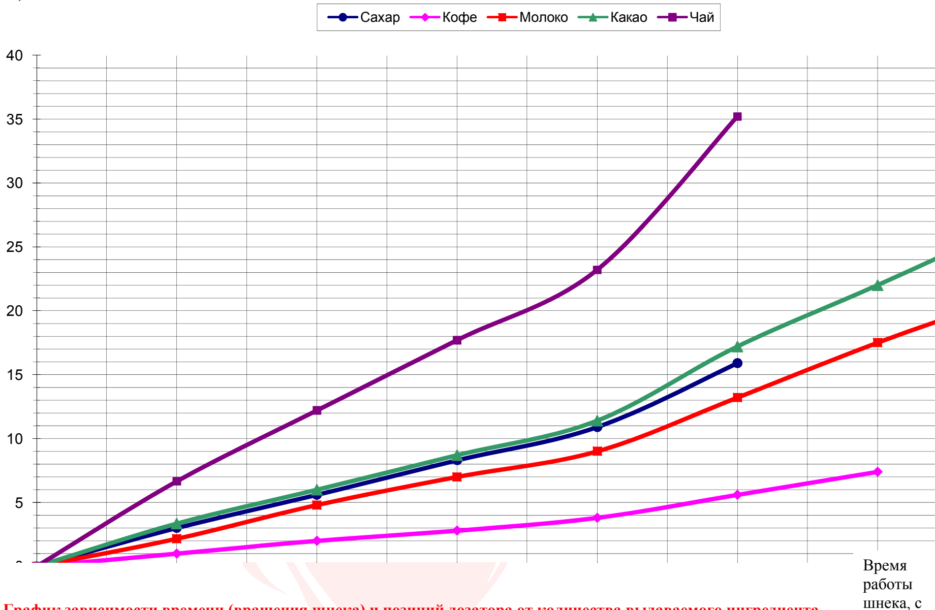
Рис 11. График зависимости времени (вращения шнека) и позиций дозатора от количества выдаваемого ингредиента
